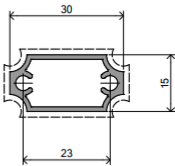
DE 1062 | 0,317 Kg/m
