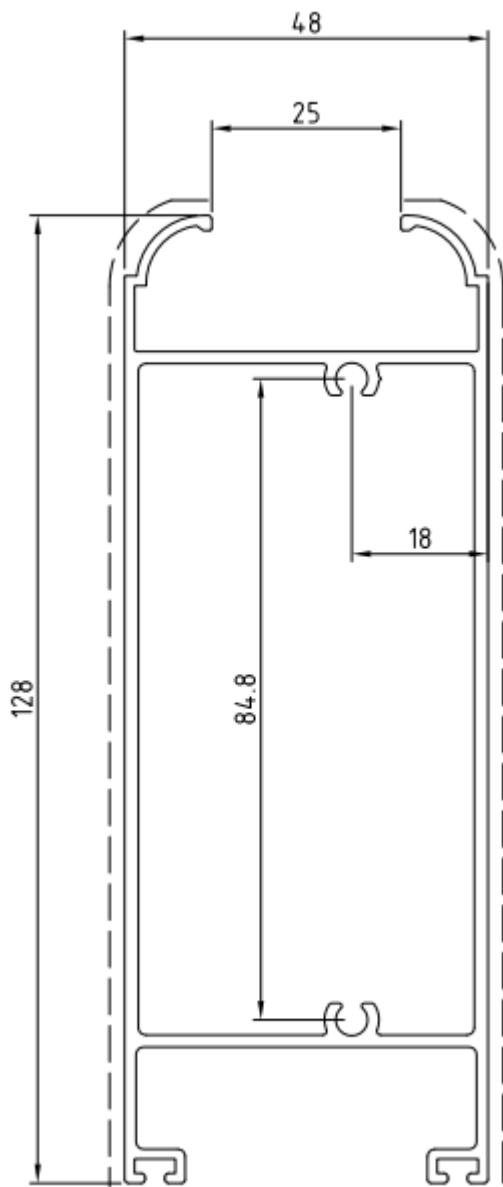
DE 1029 | 1,770 Kg/m
