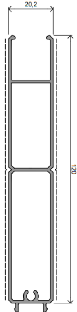
DE 1043 | 0,960 Kg/m
