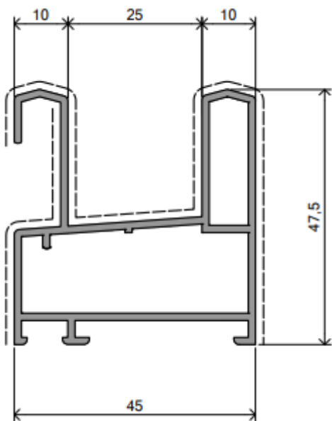
DE 1049 | 0,748 Kg/m
