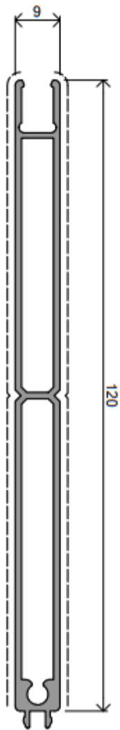
DE 1042 | 0,886 Kg/m
