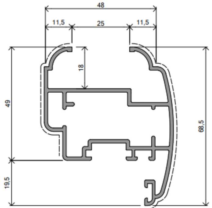
DE 1020 | 1,225 Kg/m
