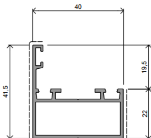
DE 1029 | 1,770 Kg/m
