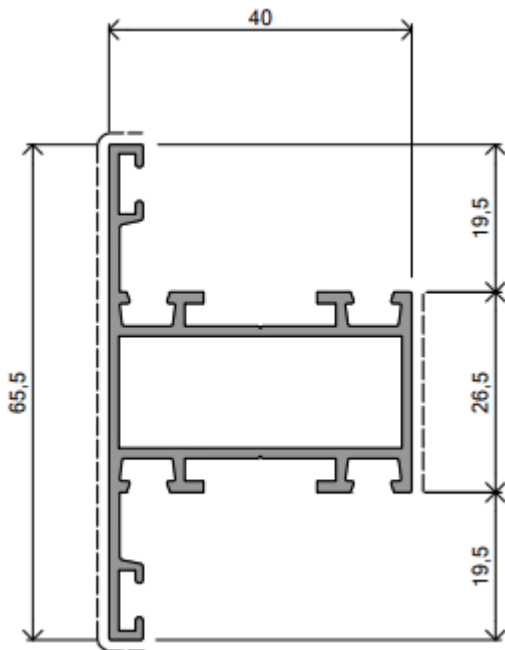
DE 1035 | 0,799 Kg/m
