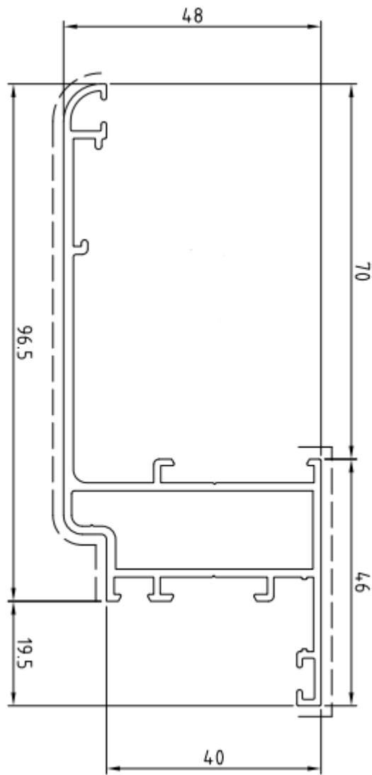
DE 1016 | 1,150 Kg/m
