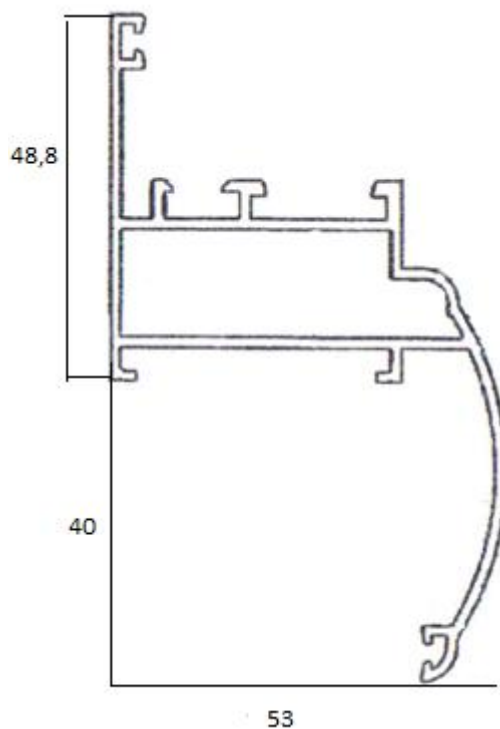
DE 1011 | 0,960 Kg/m
