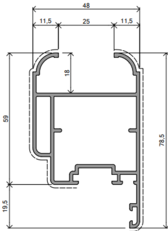
DE 1019 | 1,207 Kg/m
